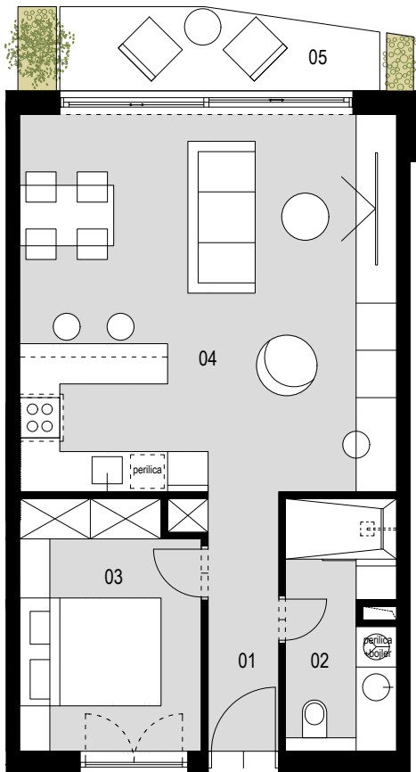
TLOCRT STANA M 1:100 S36
