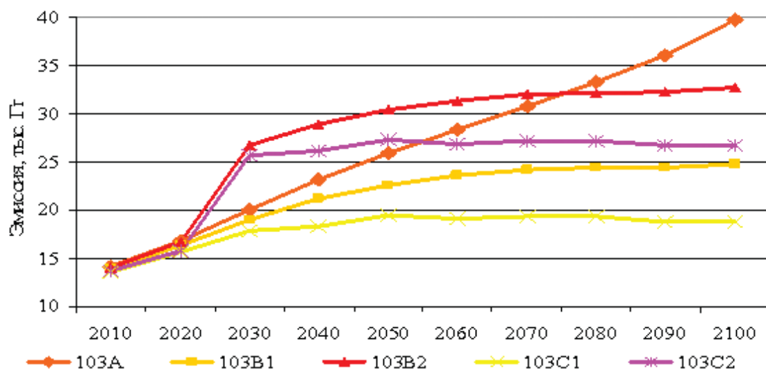
Рис. 6.5. Эмиссия ПГ в \text{CO}_2 -эквиваленте по сценариям при экономическом росте 3% в год
