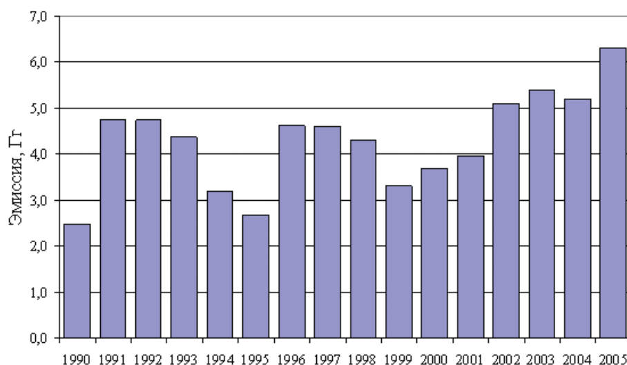
Рис. 3.42. Эмиссии НМЛОС при производстве продовольствия и напитков
