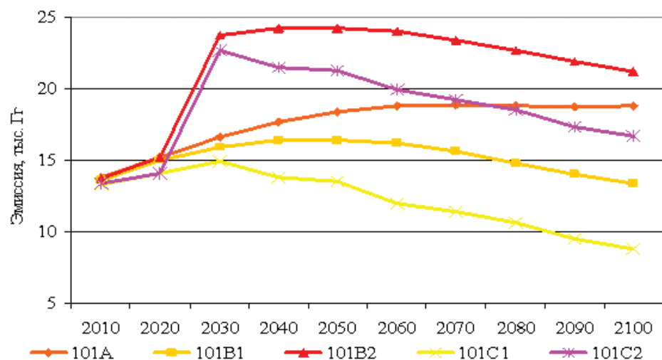
Рис. 6.3. Эмиссия ПГ в \text{CO}_2 -эквиваленте по сценариям при экономическом росте 1% в год
