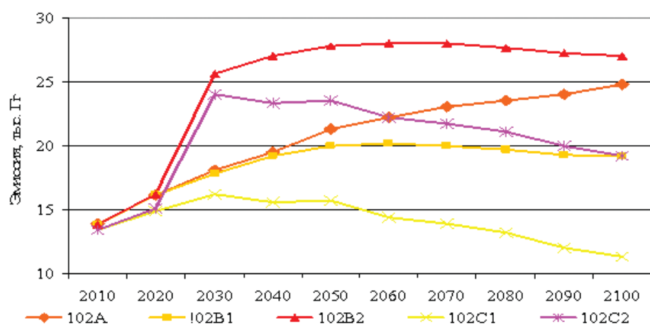
Рис. 6.4. Эмиссия ПГ в \text{CO}_2 -эквиваленте по сценариям при экономическом росте 2% в год
