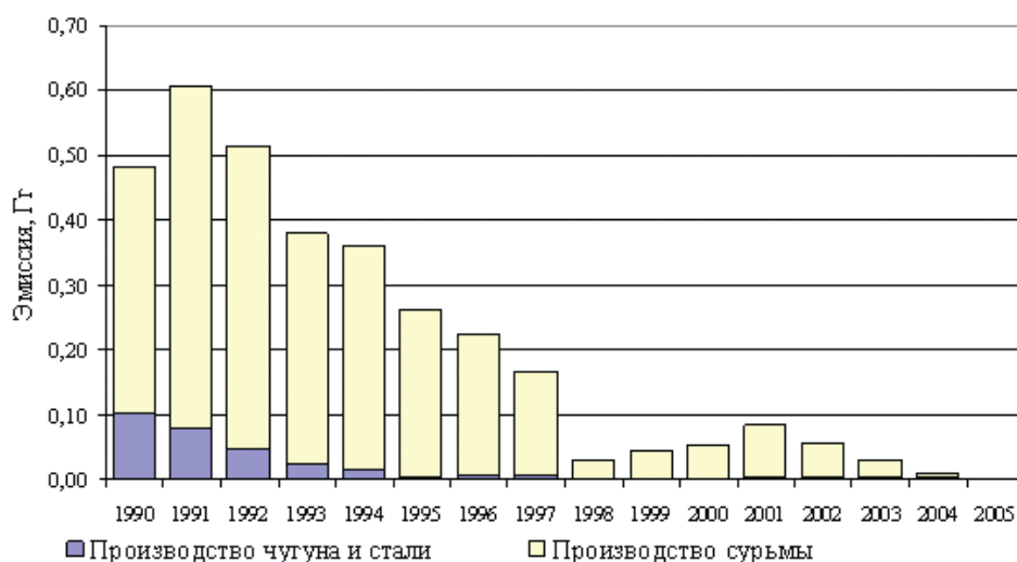
Рис. 3.39. Эмиссия оксидов азота в секторе производства металлов
