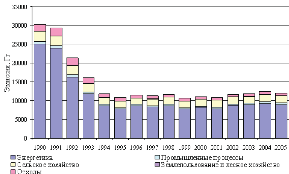
Рис. 3.2. Эмиссии суммы парниковых газов с учетом ПГП по разделам
