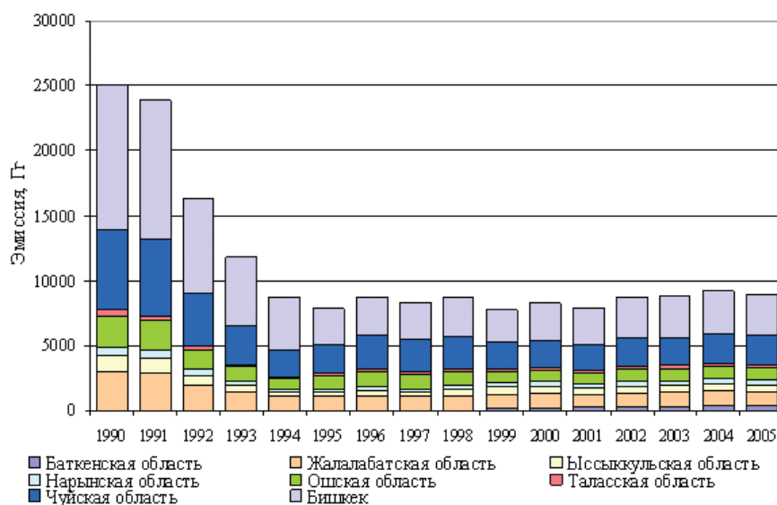
Рис. 3.68. Изменение распределения эмиссии парниковых газов (с учетом ПГП) в разделе «Энергетика» по регионам
