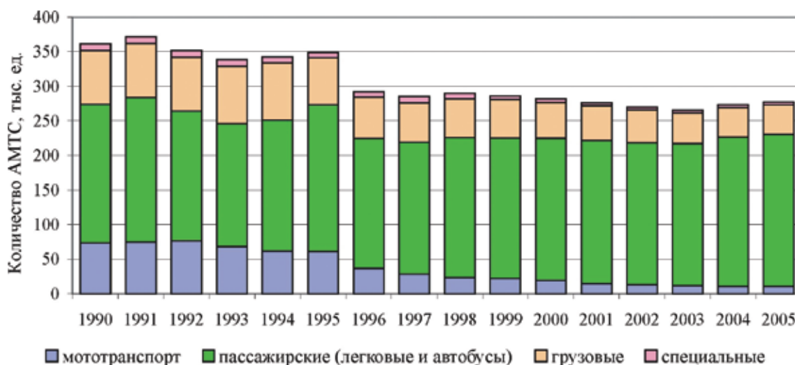
Рис. 2.14. Динамика наличных, технически исправных АМТС в республике
