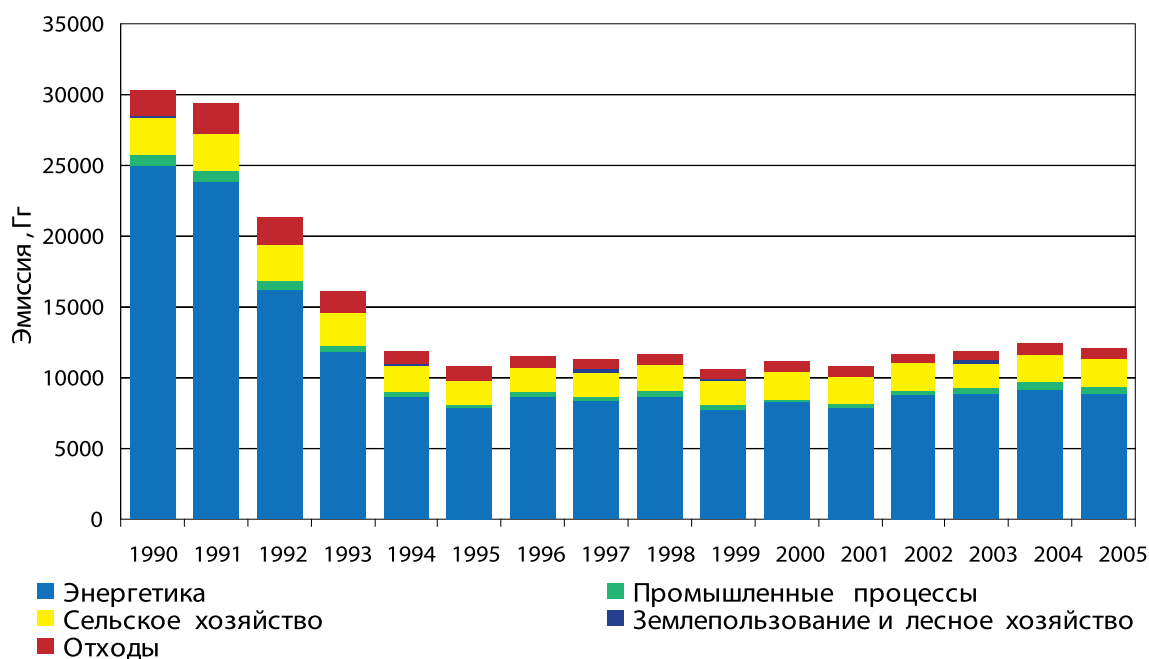
Рис. Р.5. Эмиссия суммы парниковых газов с учетом ПГП по разделам
