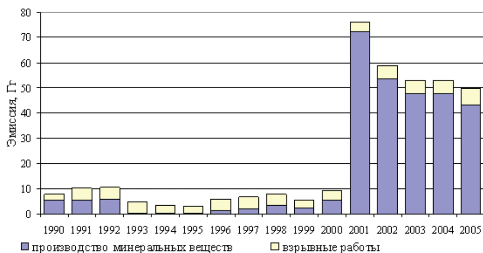
Рис. 3.31. Распределение эмиссии НМЛОС. Небольшой объем эмиссии наблюдался также и в секторе «Химическая промышленность», с максимальными значениями, не превышающими 0,02 Гг
