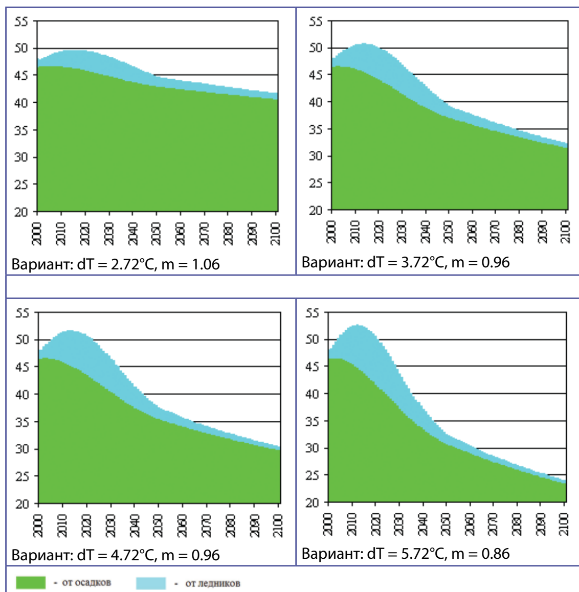
Рис. 5.4. Динамика структуры поверхностного стоке всего Кыргызстана для
