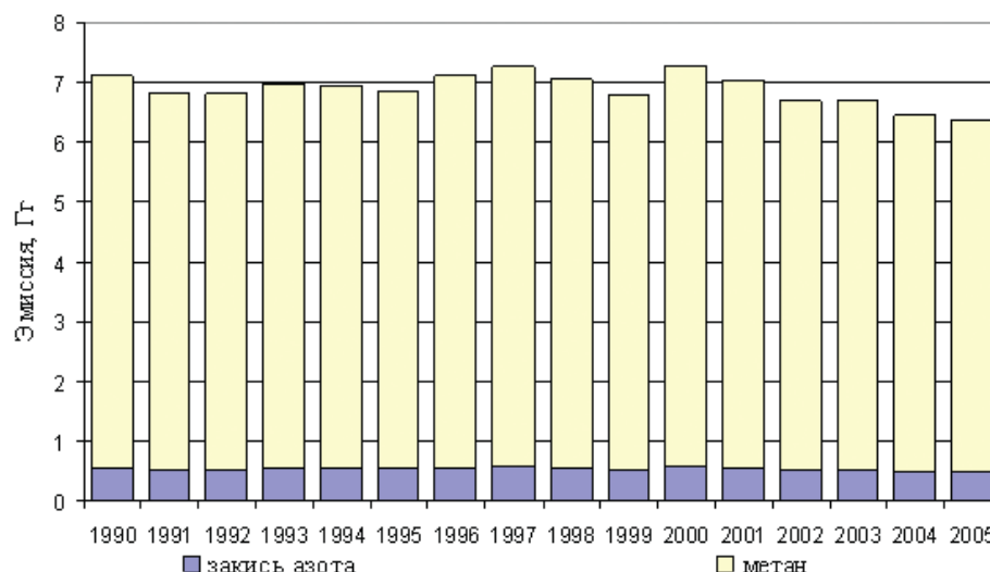
Рис. 3.57. Эмиссия парниковых газов (кроме CO 2 ) в секторе «Изменение запасов древесной биомассы» при сжигании биомассы (с учетом ППП)
