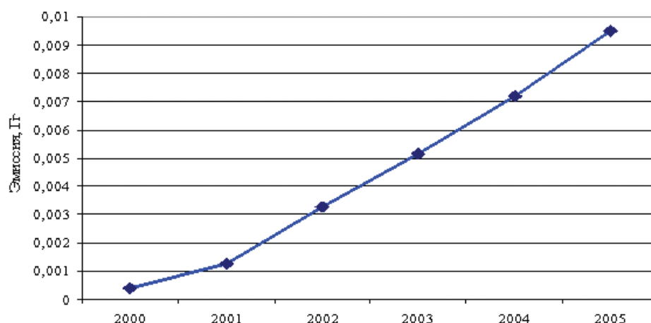
Рис. 3.44. Эмиссия ГФУ-134а при обслуживании охлаждающего оборудования
