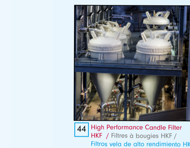
44 High Performance Candle Filter HKF / Filtrés à bougies HKF / Filtros vela de alto rendimiento HKF
