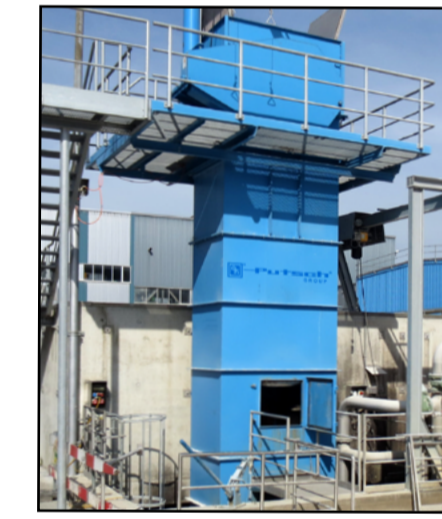
8 Belt Type Rock Catcher GSA / Épierreurs à courroies GSA / Despedrador de canchales GSA
